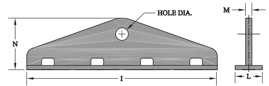
Top and Bottom Lug Plates
